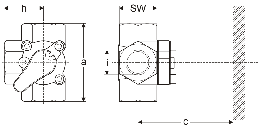
Рис. 1. Размеры V5433A
