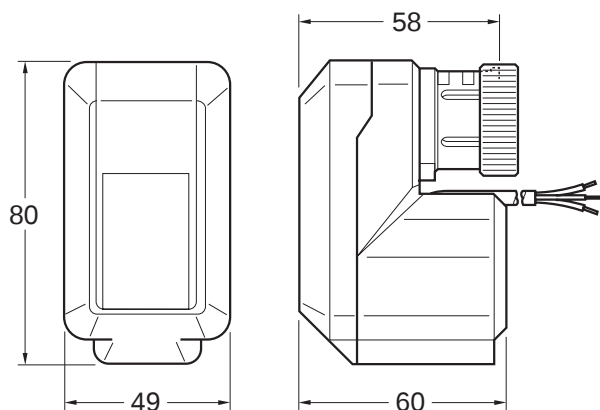
Рис.12 Тип корпуса А
